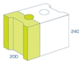
BIA-20/24-1/3e BLOK
